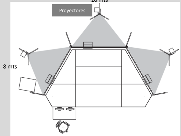
PROYECCIÓN TRASERA
